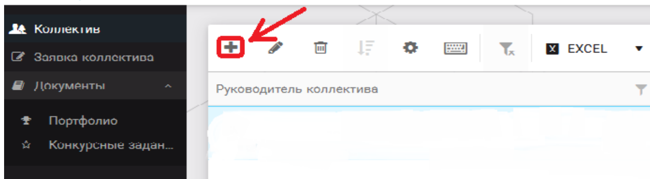
Рисунок 4 – Создание коллектива
