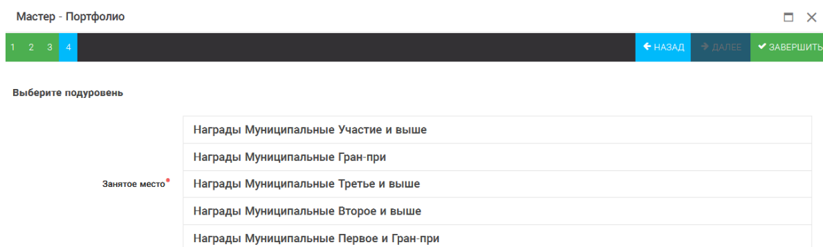
Рисунок 15 – Выбор места
