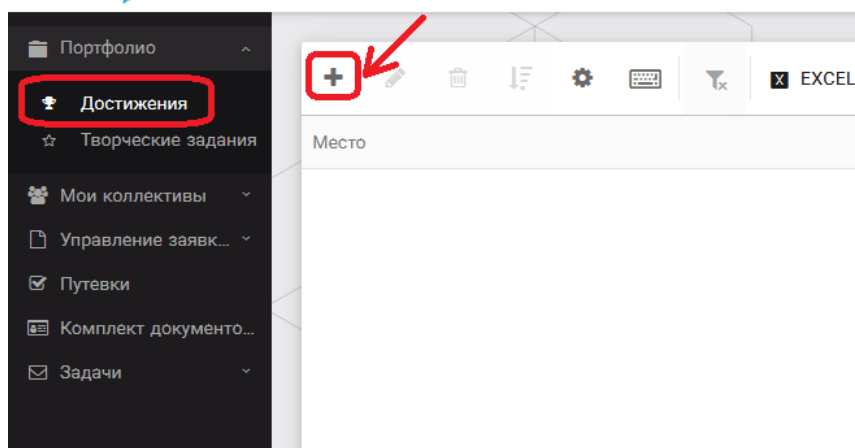
Рисунок 11 – Загрузка достижений
